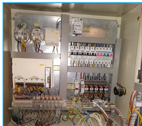
■ Výměna technologického zařízení výměňkové stanice ZŠ Husovo náměstí
