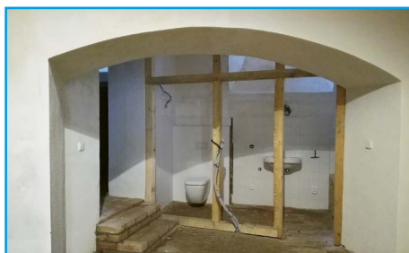
■ Zbývá provést opláštění dřevěné kostry příčky
