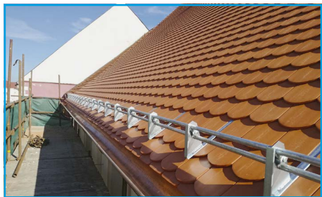
■ Zachytávač sněhu
