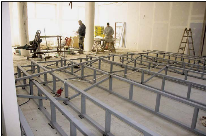
■ Ocelová konstrukce pódia v malém sále Záložna je připravena pro zaklopení OSB deskami
