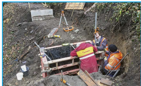
■ Instalace bednění pro základovou patku nového mostku
